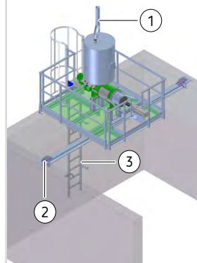
Podest mit Mauerauflage
