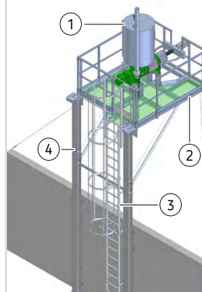
Podest mit Hintereinstieg an Stützmauer
