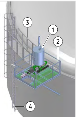
Podest mit Seiteneinstieg links an einem Gärrestlagerbehälter
